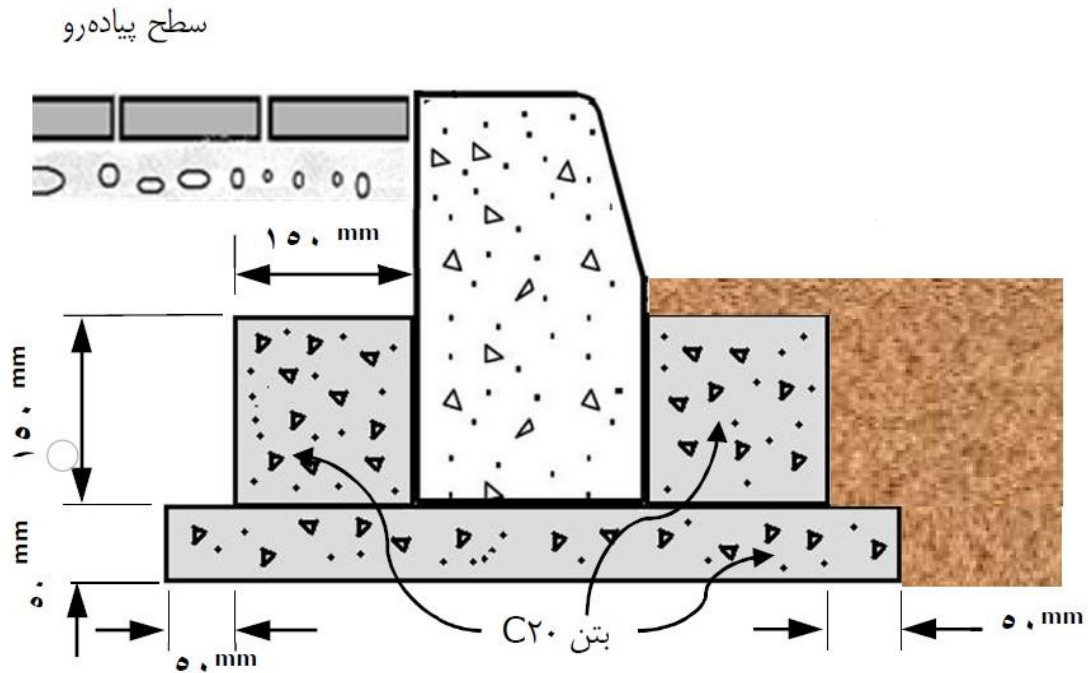
جزئیات نصب جداول قائم (تک جدول) - تیپ A
